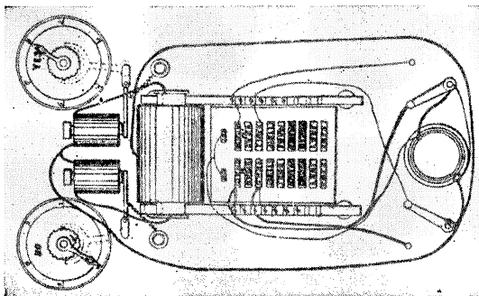
Генератор Эдисона нижним расположением якоря.
